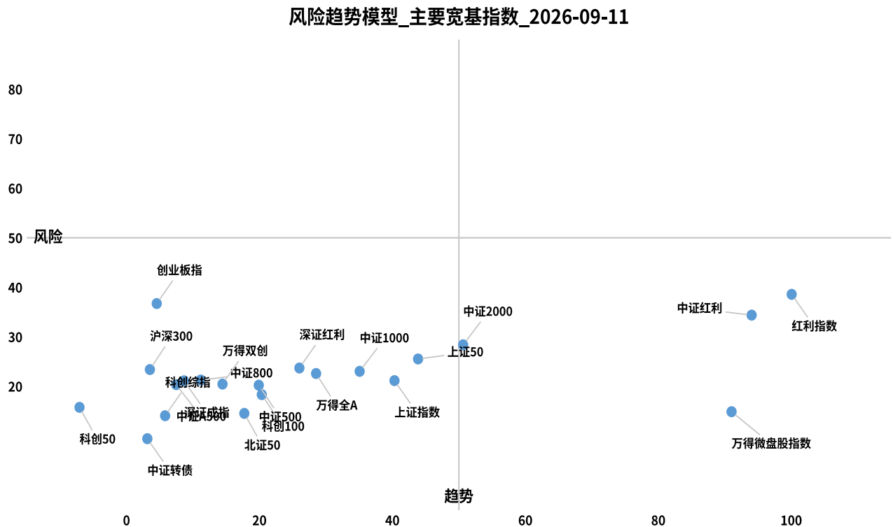
图7: 2026年9月11日主要宽基指数风险趋势模型综合图
