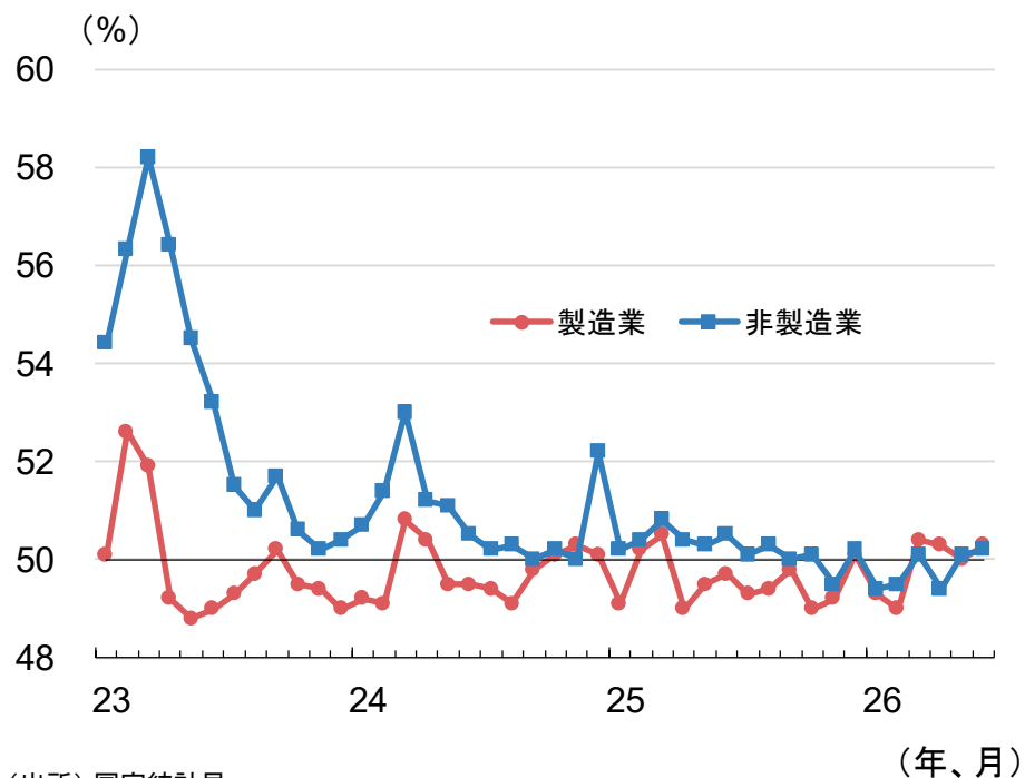
PMI
