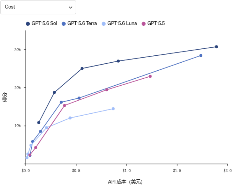
GeneBench v1
