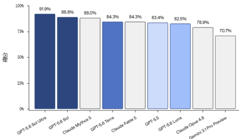
TerminalBench 2.1
