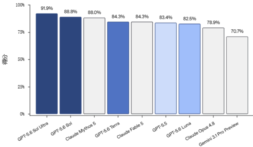
TerminalBench 2.1
