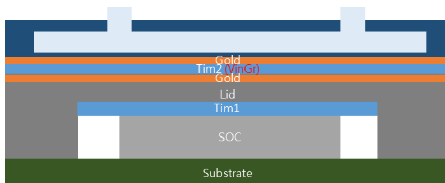
圖 3：鍍金水冷板示意圖
