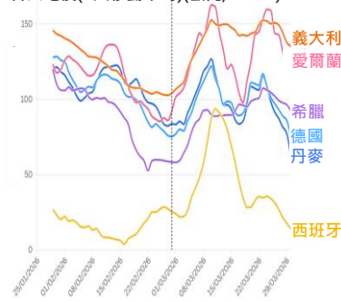
各國電價(7天移動平均)(歐元/MWh)
