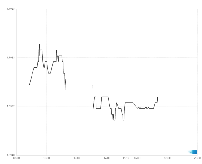
附图 17: 8 月 7 日 10Y 国债活跃券收益率震荡下行
