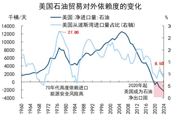
图3：页岩油革命让美国降低对外石油依赖度
