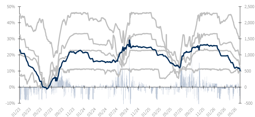
Biểu đồ 7. Tỷ lệ cao hơn mực nước chết và lưu lượng ròng tại hồ thủy điện Thác Bà
