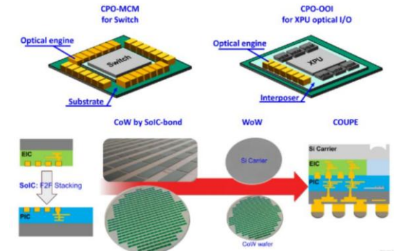
圖三：台積電 COUPE 平台
