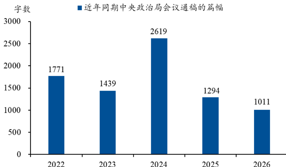
图 1：本次会议通稿是近年来同期最短的
