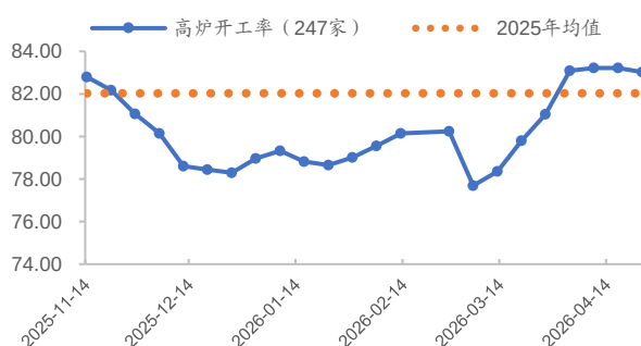
图1 高炉开工率 (%)
