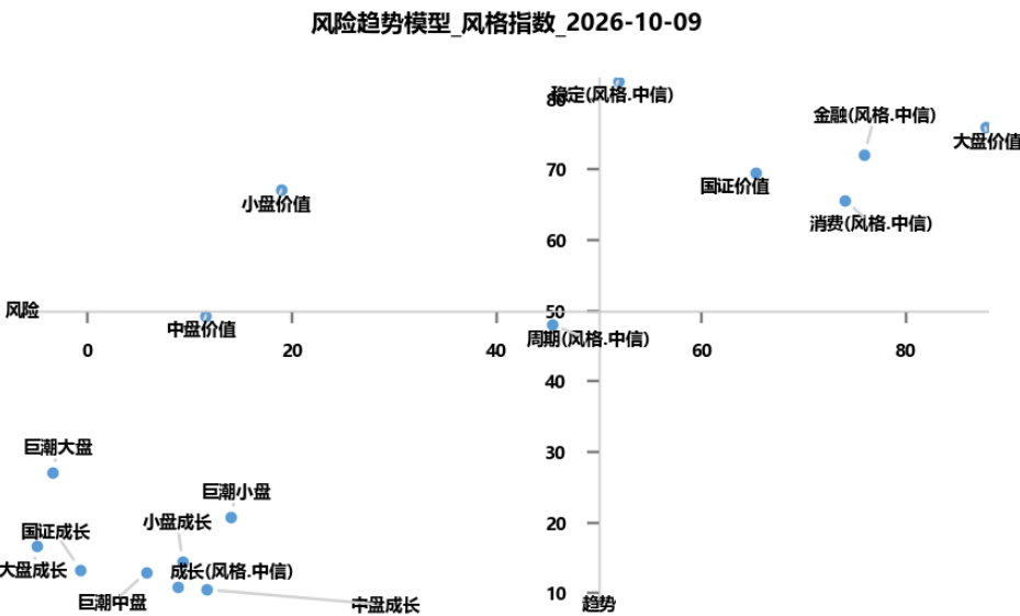
图9：2026 年 10 月 9 日风格指数风险趋势模型综合图
