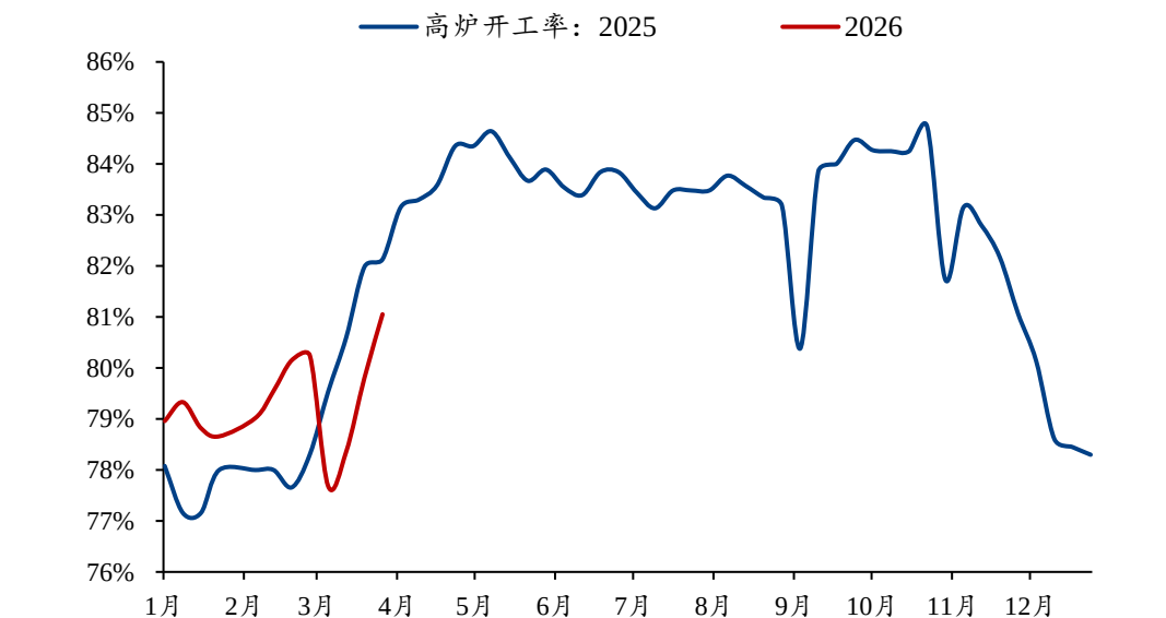
图表3：2025 年和 2026 年高炉开工率对比
