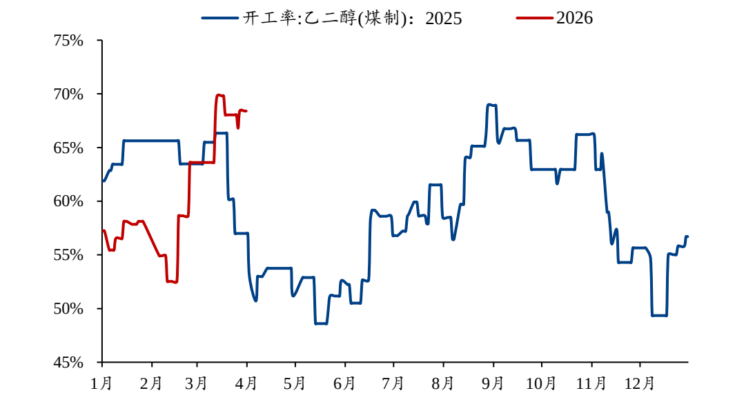
图表9：3月以来，煤制乙二醇开工率大幅上升
