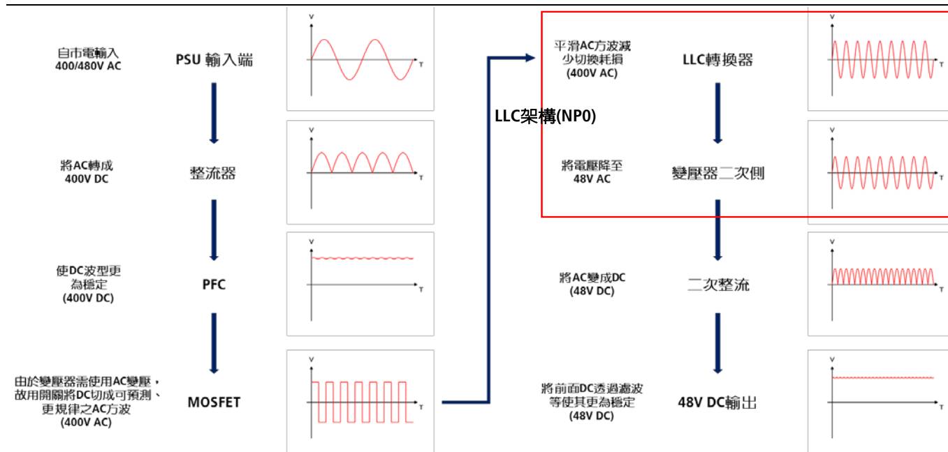
圖 1：現行 PSU 架構內電力傳輸路徑
