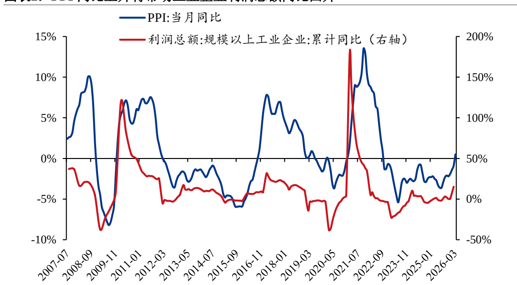
图表2：PPI 同比上升将带动工业企业利润总额同比回升
