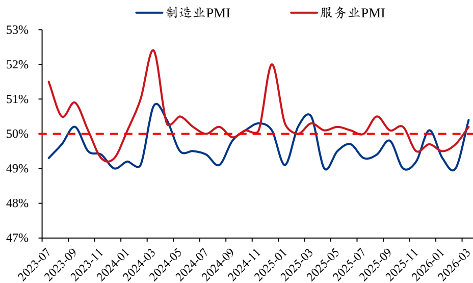
图表4：3月制造业和服务业 PMI 重回扩张区间
