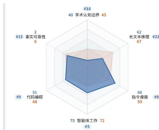
GLM 5.1
