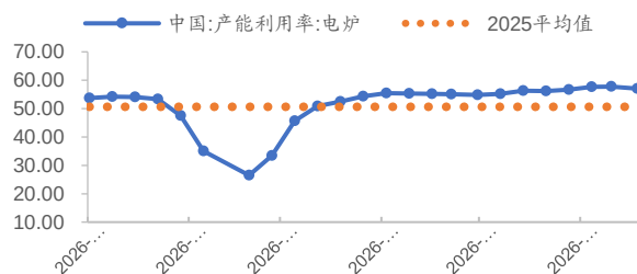
图23 电炉产能利用率 (%)
