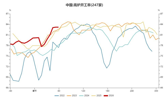
图 30：高炉开工率持平前周
