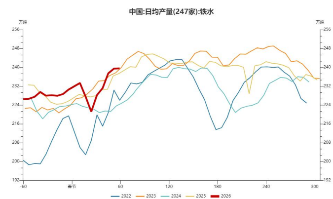
图 32：日均铁水产量持平前周
