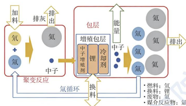
图表 44：聚变主循环原理示意图
