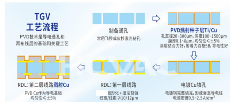
图.镀铜与通孔属于玻璃基板的核心工艺
