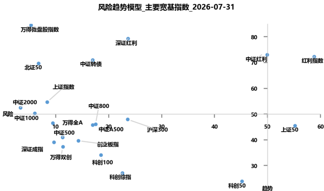
图7：2026 年 7 月 31 日主要宽基指数风险趋势模型综合图
