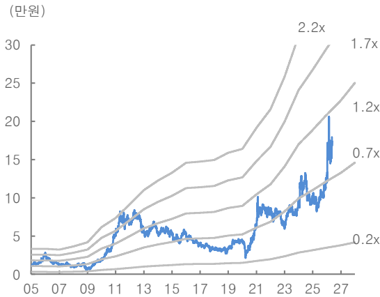
그림 4. 기아 12개월 선행 PBR Band
