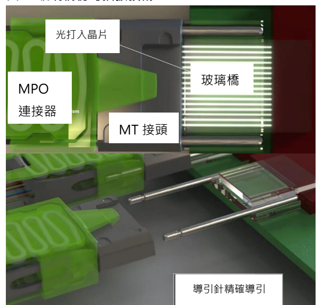
圖 4 玻璃橋仿可插拔技術
