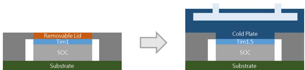
圖 5：Removeable Lid 可望在 Rubin Ultra 中採用
