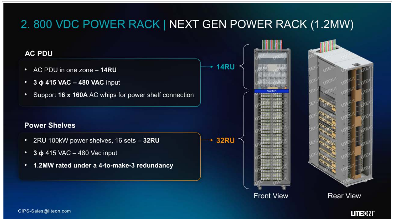
圖 7：光寶科 HVDC 機櫃設計原型 (GTC 大會)
