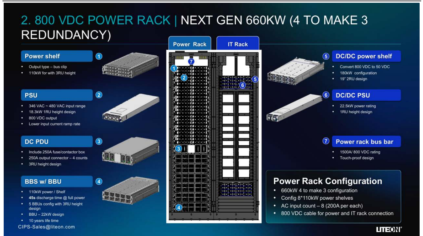
圖 6：光寶科 HVDC 機櫃設計原型 (GTC 大會)
