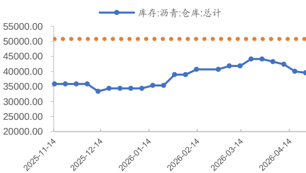
图22 沥青库存 (吨)
