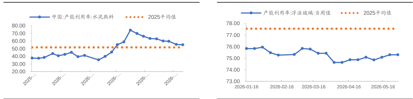
图25 水泥熟料产能利用率（%）
