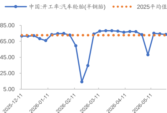
图12 半钢胎开工率 (%)
