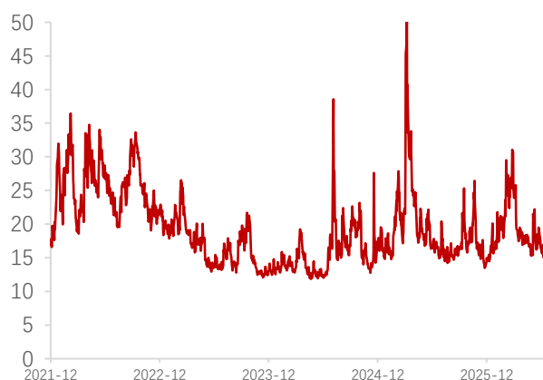
图 18: VIX
