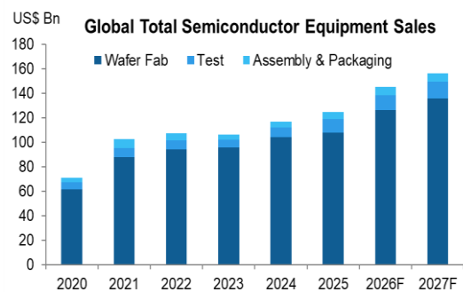
圖 5：2026/27 年半導體設備銷售 YoY +16.2%/+7.6%
