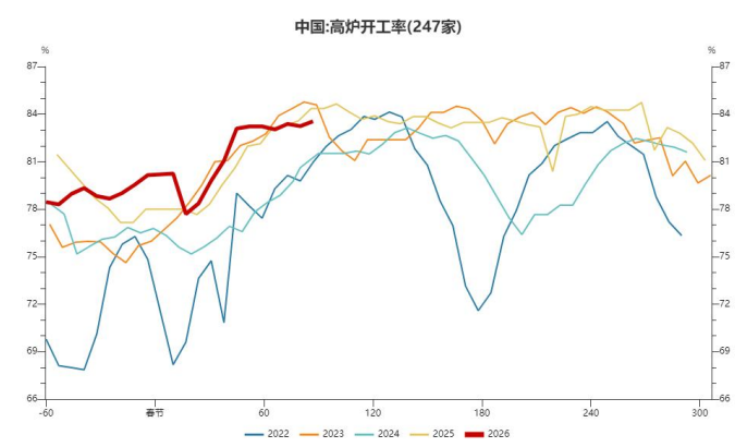
图 10：高炉开工率上升
