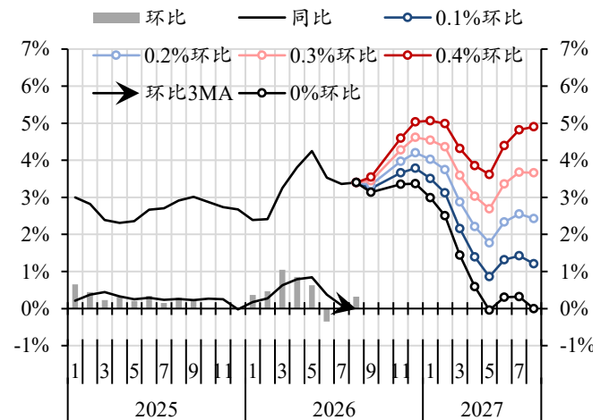
图15: 不同环比路径下美国 CPI 同比走势
