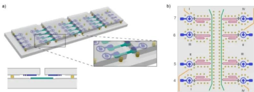
图 7: Rigetti 多核架构示意图
