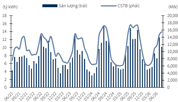
Biểu đồ 10. Sản lượng và công suất trung bình thủy điện toàn quốc đến T08/26
