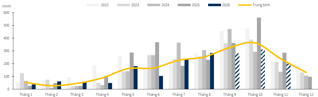
Biểu đồ 9. Dự báo lượng mưa cả nước trong tháng 09/26-11/26
