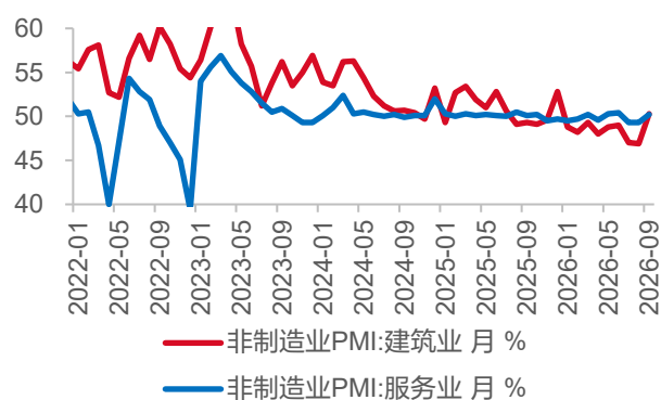
图9 建筑业、服务业 PMI，%
