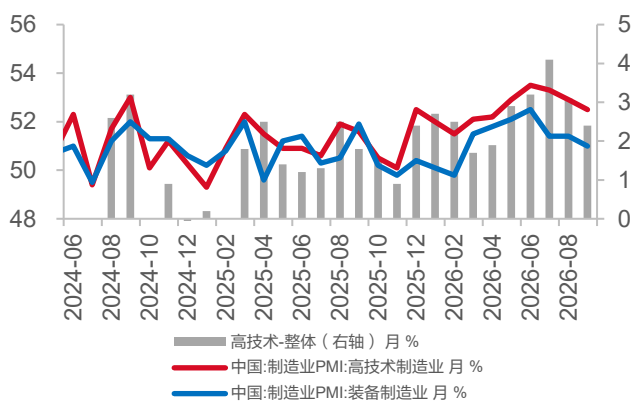
图6 高技术制造业、装备制造业 PMI，%
