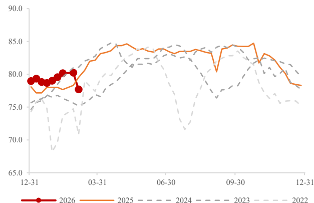
图 26：高炉开工率（%）
