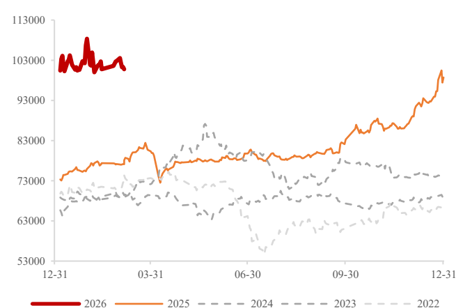
图 24：阴极铜（元/吨）
