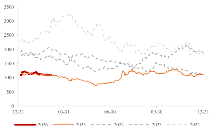
图 22：焦煤（元/吨）
