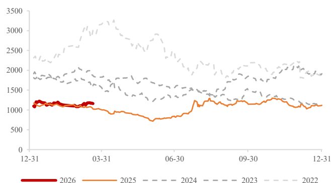
图 28：焦煤（元/吨）
