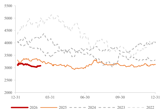
图 23：螺纹钢（元/吨）
