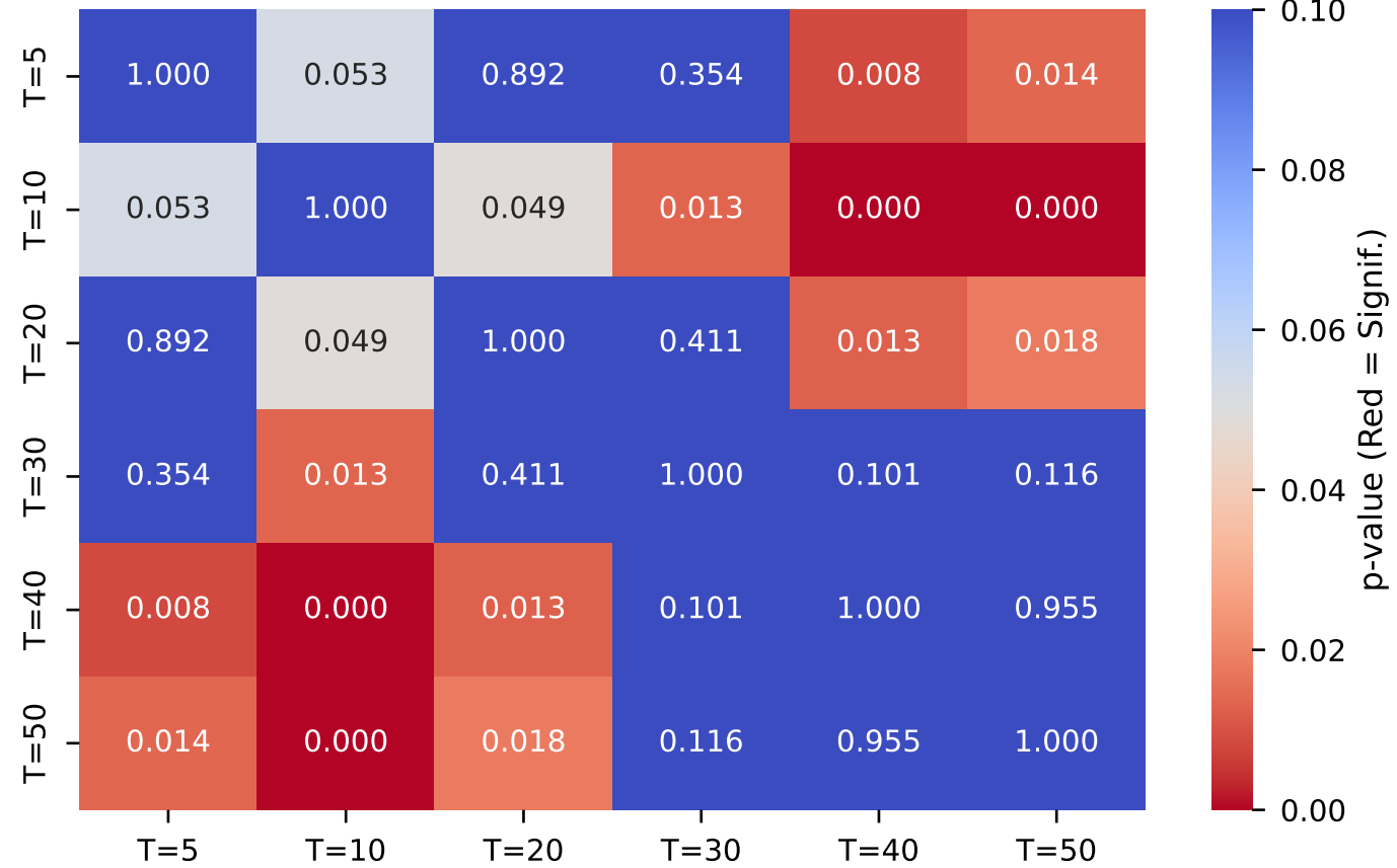
FFSNN
