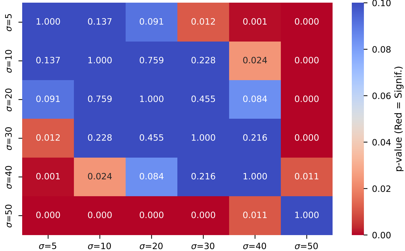
CSNN
