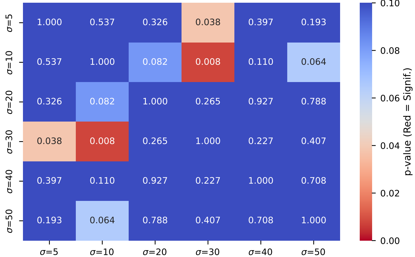
FFSNN
