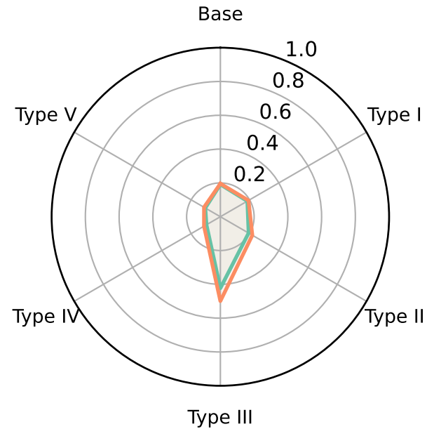
PR-AUC
