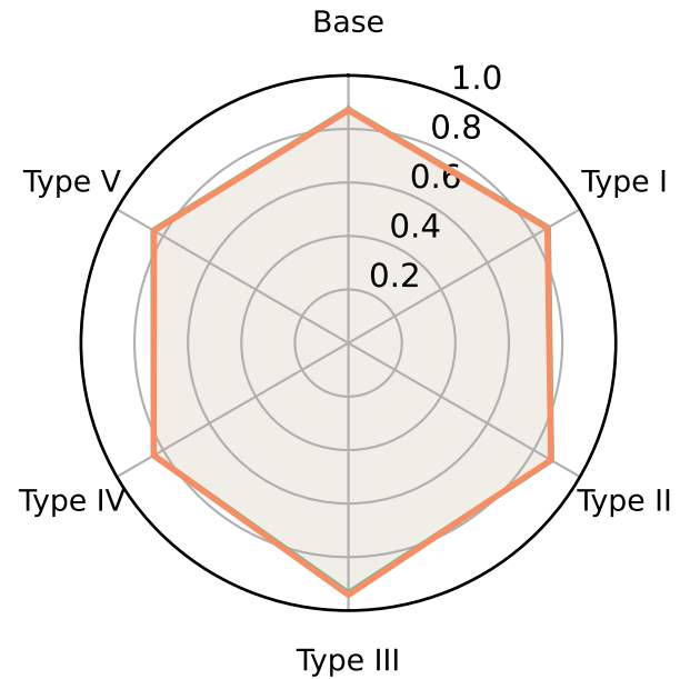
ROC-AUC
