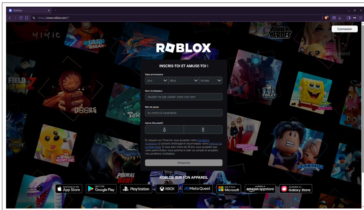
Fig. 1. – Page d'inscription.
