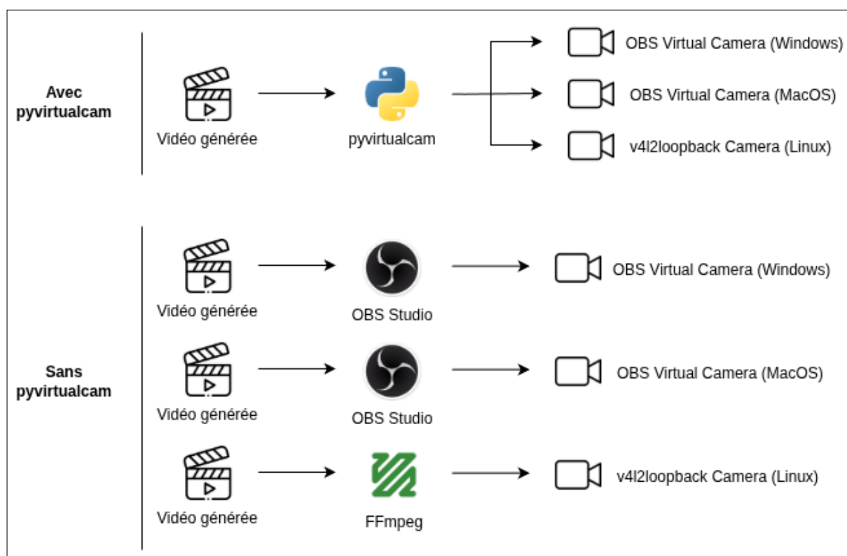
Fig. 1. – Comparaison avec pyvirtualcam et sans pyvirtualcam pour rediriger un flux vidéo vers une caméra virtuelle.
