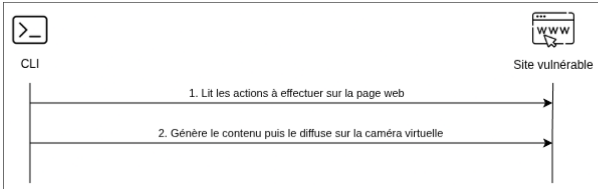
Fig. 9. – Le démonstrateur lit les instructions du site vulnérable, génère le contenu demandé, puis le diffuse sur la caméra virtuelle.
