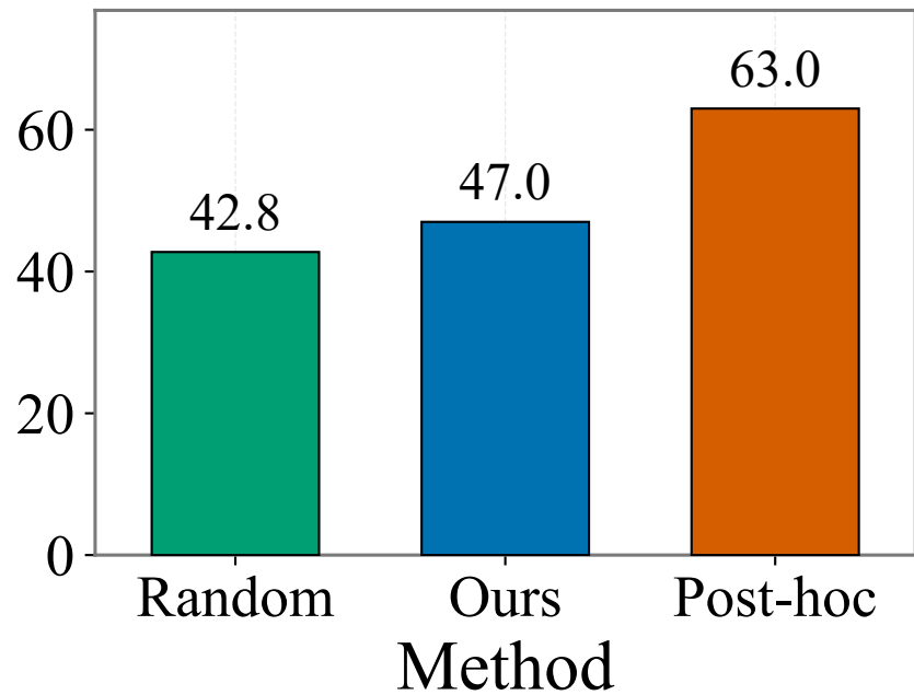
CIFAR-100 / VGG11
