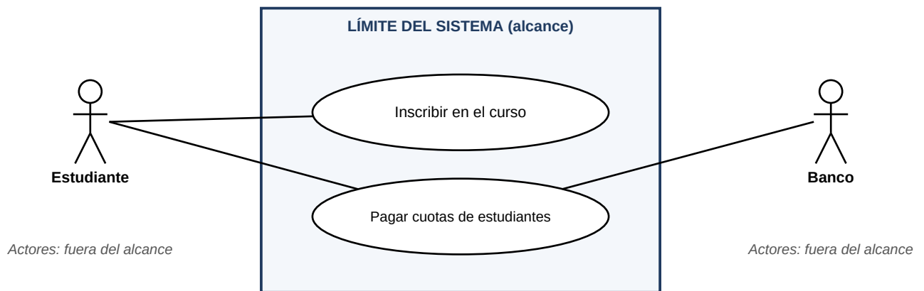
Figura 1. Alcance en un diagrama de casos de uso (esquema ilustrativo). Las líneas de comunicación que cruzan el límite son las que definen el alcance.
