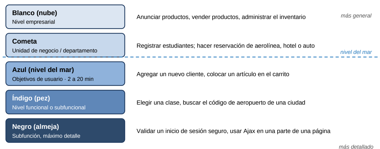
Figura 3. Niveles de los casos de uso según Cockburn (esquema propio a partir del texto)
