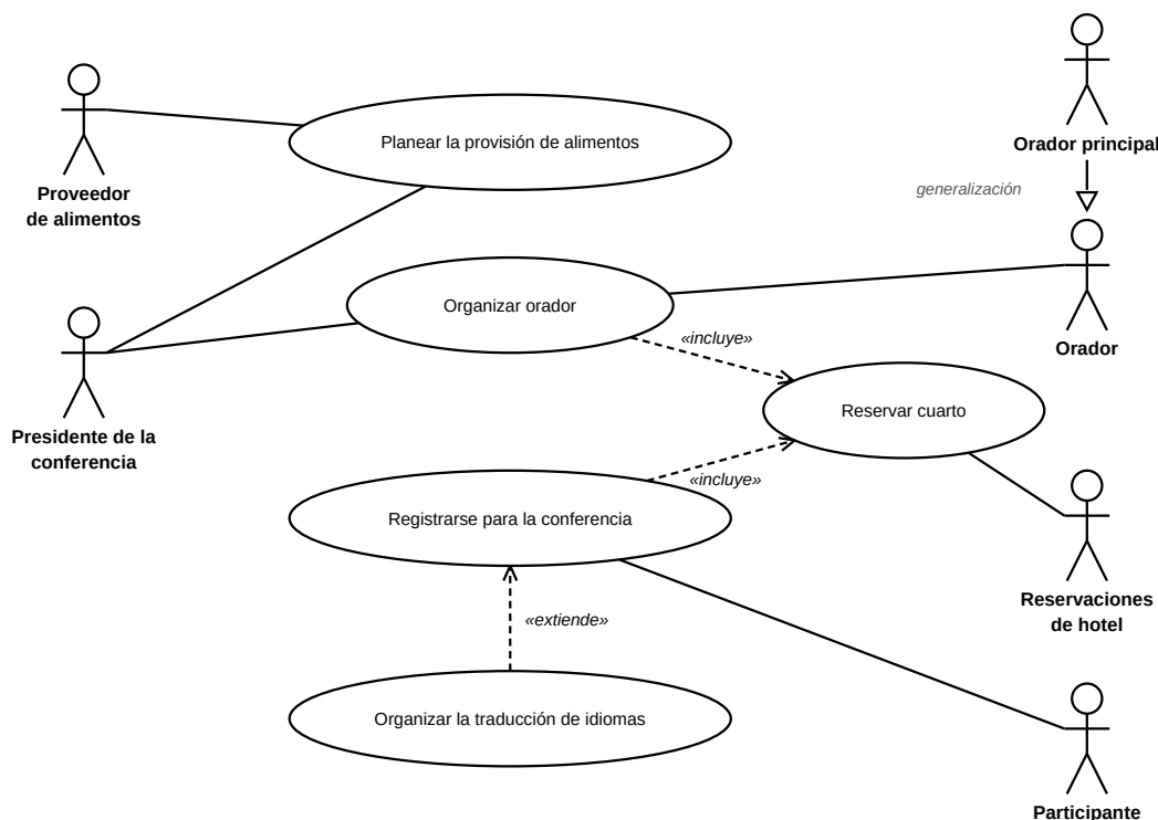
Figura 2. Diagrama de casos de uso para planear una conferencia (redibujado a partir de la figura 2.15; las líneas de comunicación entre actores y casos son una interpretación del texto)
