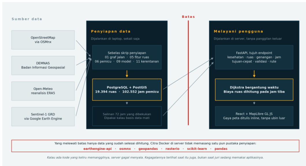
Gambar 1. Arsitektur sistem. Empat sumber terbuka di kiri masuk ke dunia penyiapan yang berjalan di laptop; hasilnya mengendap di basis data dan satu potret beku. Dunia melayani di kanan hanya membaca keduanya. Garis merah menandai batas yang tidak dilewati kode pipeline, dan pita di bawah menyebutkan pustaka mana saja yang sengaja tidak dipasang di server.
