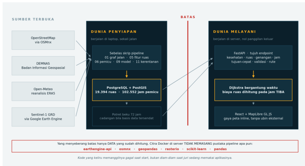
Gambar 9 — Arsitektur sistem. Empat sumber terbuka di kiri masuk ke dunia penyiapan yang berjalan di laptop; hasilnya mengendap di basis data dan satu potret beku. Dunia melayani di kanan hanya membaca keduanya. Garis merah menandai batas yang tidak dilewati kode pipeline, dan pita di bawah menyebut pustaka mana saja yang sengaja tidak dipasang di server.
