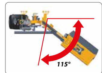
Hydraulische Anfahrtsicherung mit Überdruckventil (Schützt Auslegerarme im Fall von Hindernissen). Seguridad hidráulica en la rotación con válvula de presión máxima (protección de brazos en caso de obstáculos).
