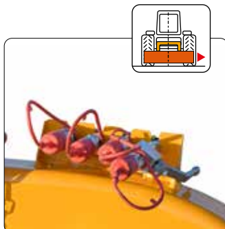
Hahn für die Hydrauliksperrung beim Transport, manuell einzulegen (keine Ketten, keine Bügel). Llave de bloqueo hidráulico para el transporte, inserción manual (sin cadenas y sin bridas).
