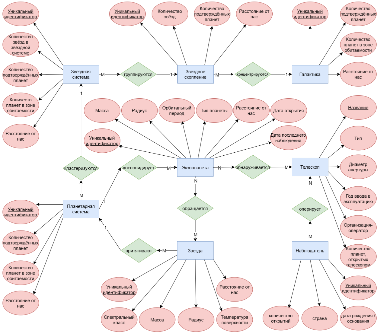
Рис. 1: ER-диаграмма
