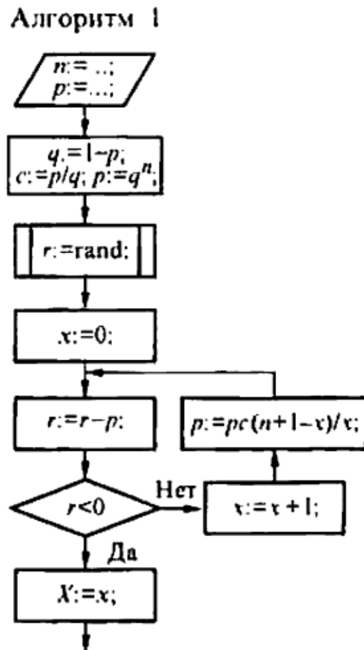
Рис. 1: Блок-схема алгоритма генерации биномиально распределённой случайной величины.
