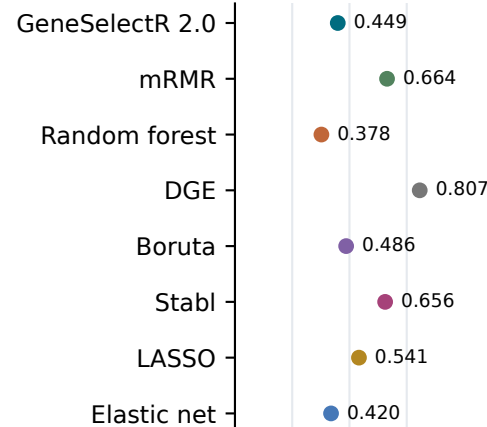
SOS-ALL
