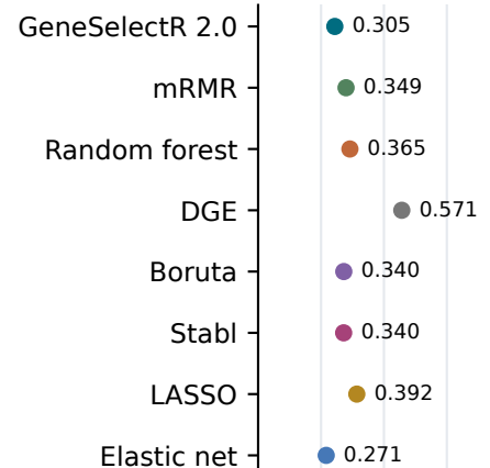
SOS-ALL
