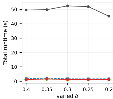
(d) Retail (fixed \gamma=0.01\% )
