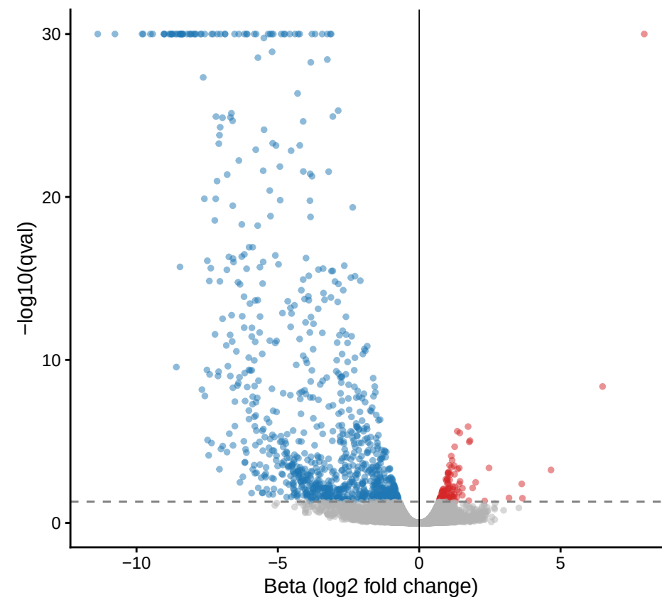
mst7 vs MST7PM | 24H
