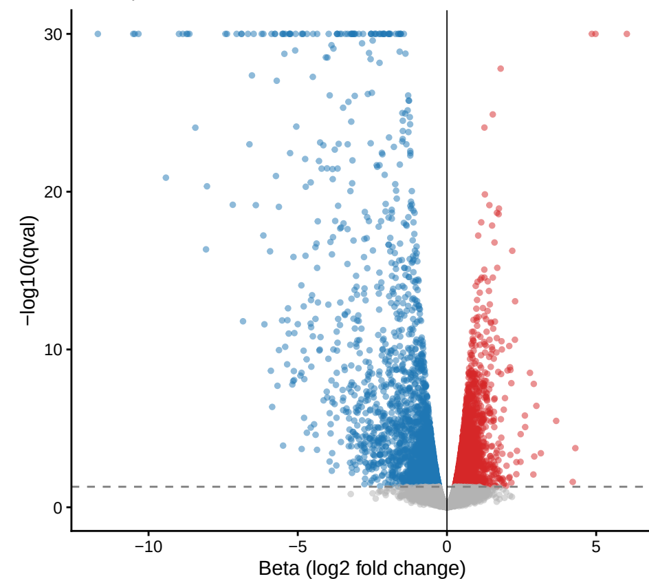
mst7 vs MST7PM | 4H
