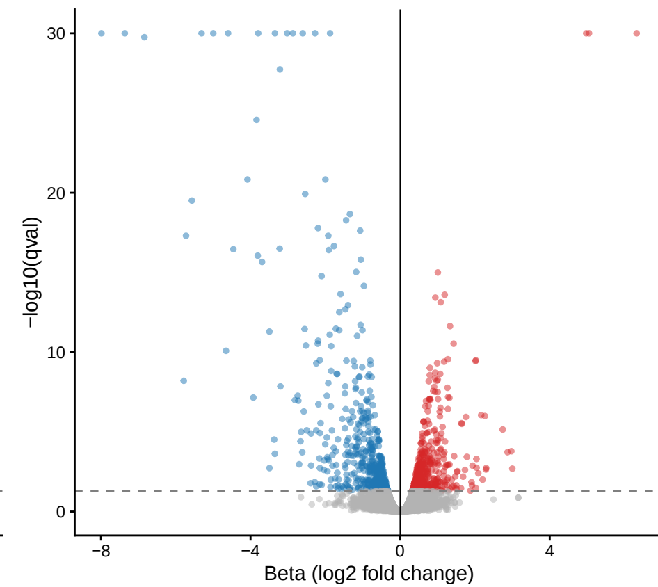
mst7 vs MST7PM | 2H
