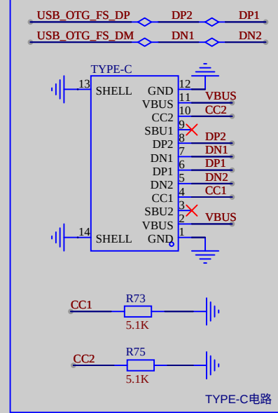
TYPE-C电路
