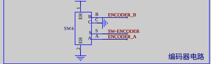
编码器电路
