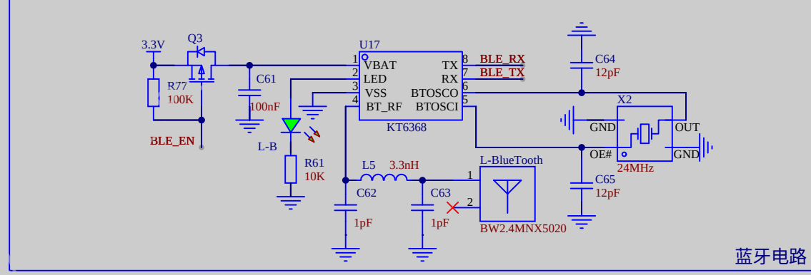
蓝牙电路
